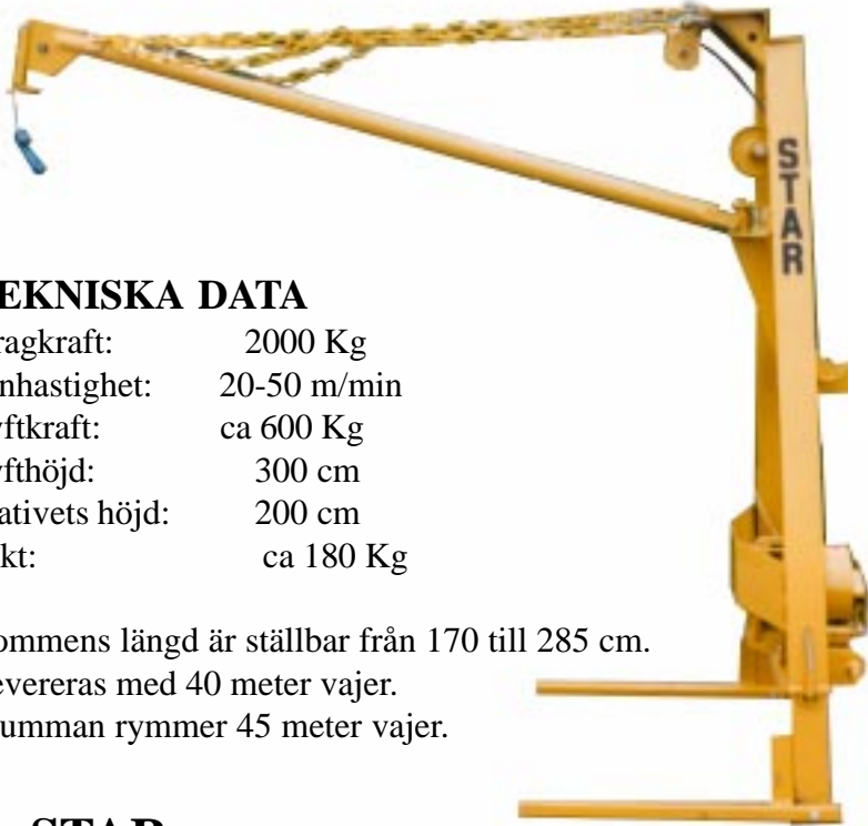
Hydraulinsvågning av bom.
